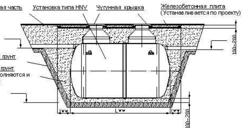
МОНТАЖ УСТАНОВКИ HNV ПОД ПРОЕЗЖЕЙ ЧАСТЬЮ
